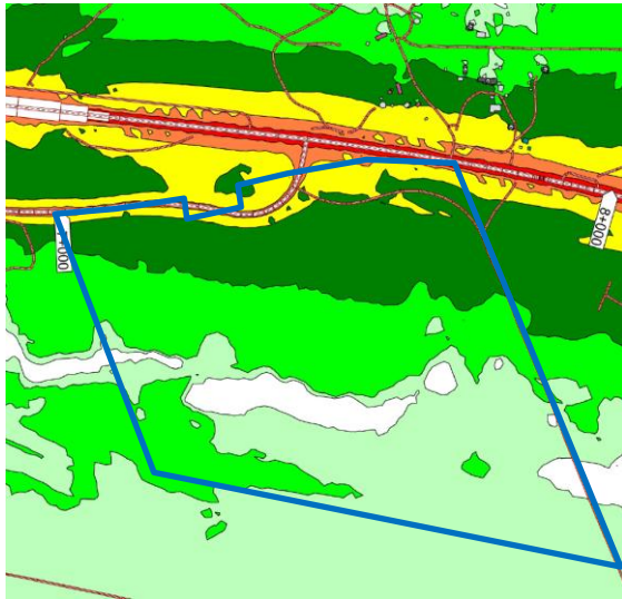
17. Tieliikenteen aiheuttama yöajan keskiäänitaso, yleissuunnitelmaratkaisu (v.2050) suunnittelualueella. © Zenner Oy 2025.
