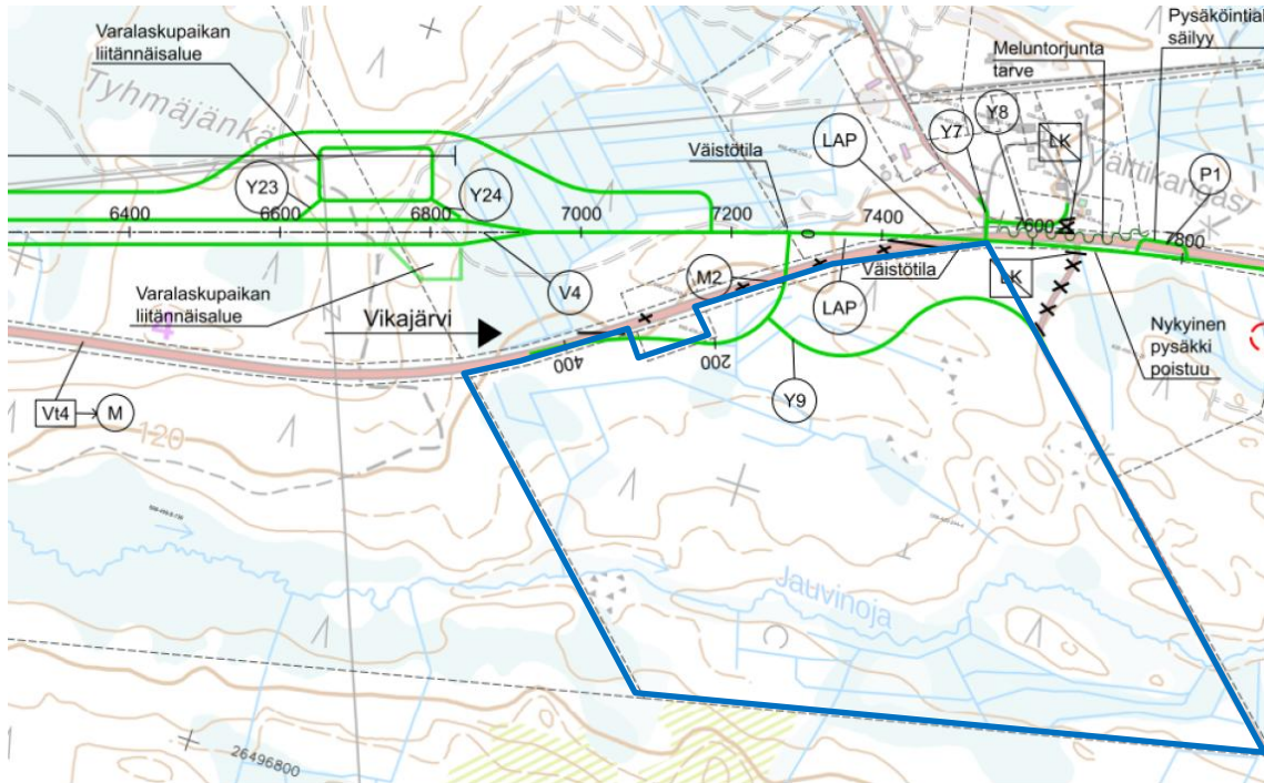
11. Ote Vt 4 uutta linjausta koskevasta Napapiiri-Apukka yleissuunnitelmasta ja suunnittelualue (sineellä). © Lapin elinvoimakeskus, 4/2026
