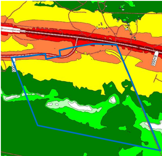
16. Tieliikenteen aiheuttama päiväjän keskiäänitaso, yleissuunnitelmaratkaisu (v.2050) suunnittelualueella. © Zenner Oy 2025.
