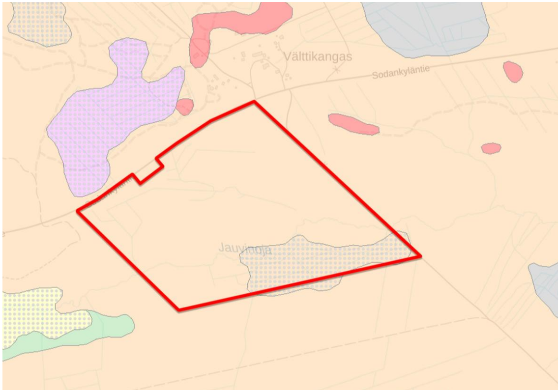
7. Alueen maaperä. © Maankamara, GTK 4/2026
