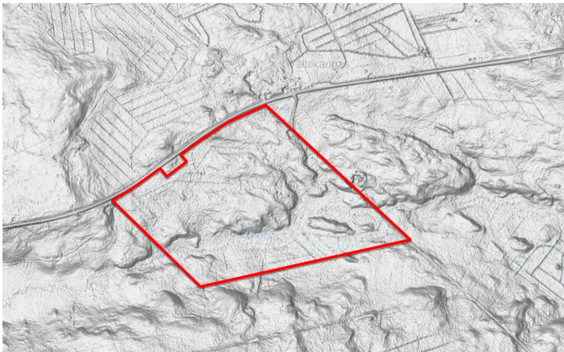
8. Korkeusmalli. © Maankamara, GTK 4/2026
