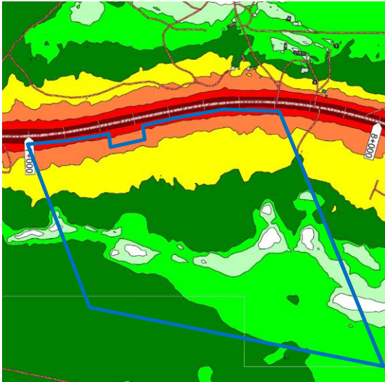
14. Tieliikenteen aiheuttama päiväjän keskiäänitaso (nykytilanne) suunnittelualueella. © Zenner Oy 2025.
