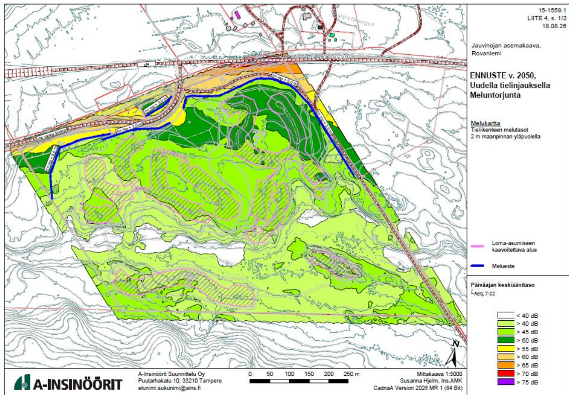
18. Ennuste v.2050, meluntorjunta uudella tielinjauksella. © A-Insinöörit Oy 2026.
