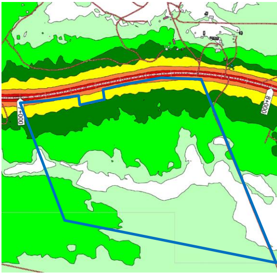
15. Tieliikenteen aiheuttama yöajan keskiäänitaso (nykytilanne) suunnittelualueella. © Zenner Oy 2025.
